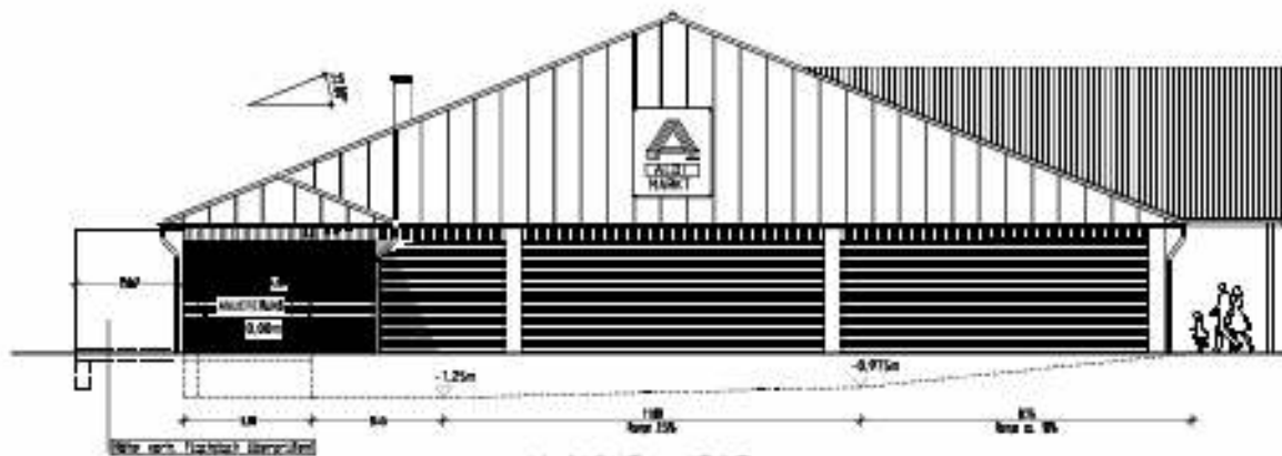
ANSICHT WEST
