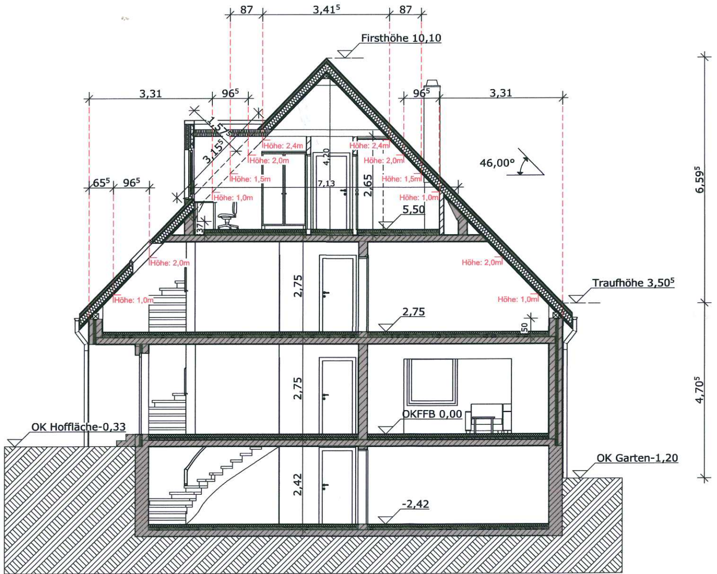
Schnitt A-A
