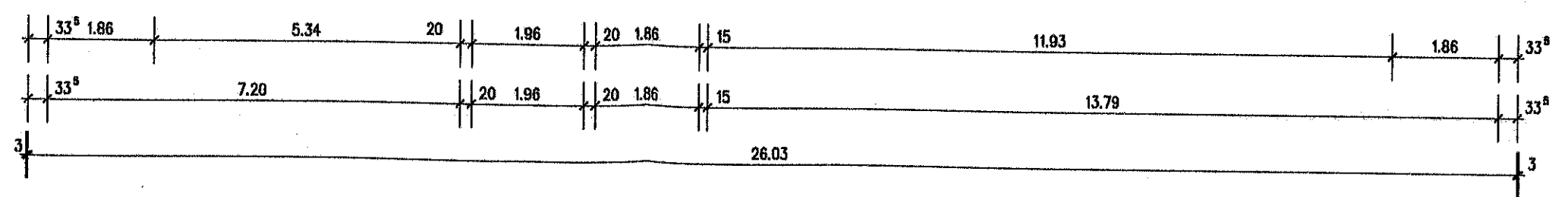
Schnitt A-B
